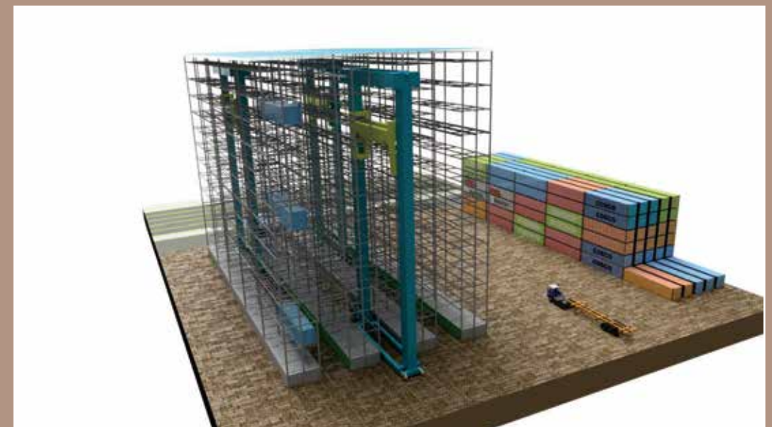
蜂窝式自动化堆场
