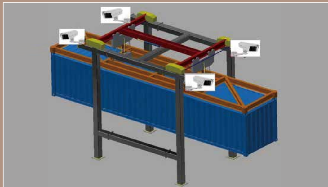
集卡自动化称量系统
